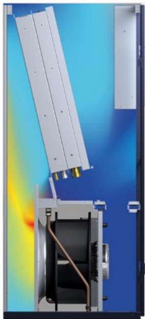
Mejores resultados de conducción de aire y funcionamiento más eficiente del sistema de aire acondicionado; el análisis se llevó a cabo con CFD
